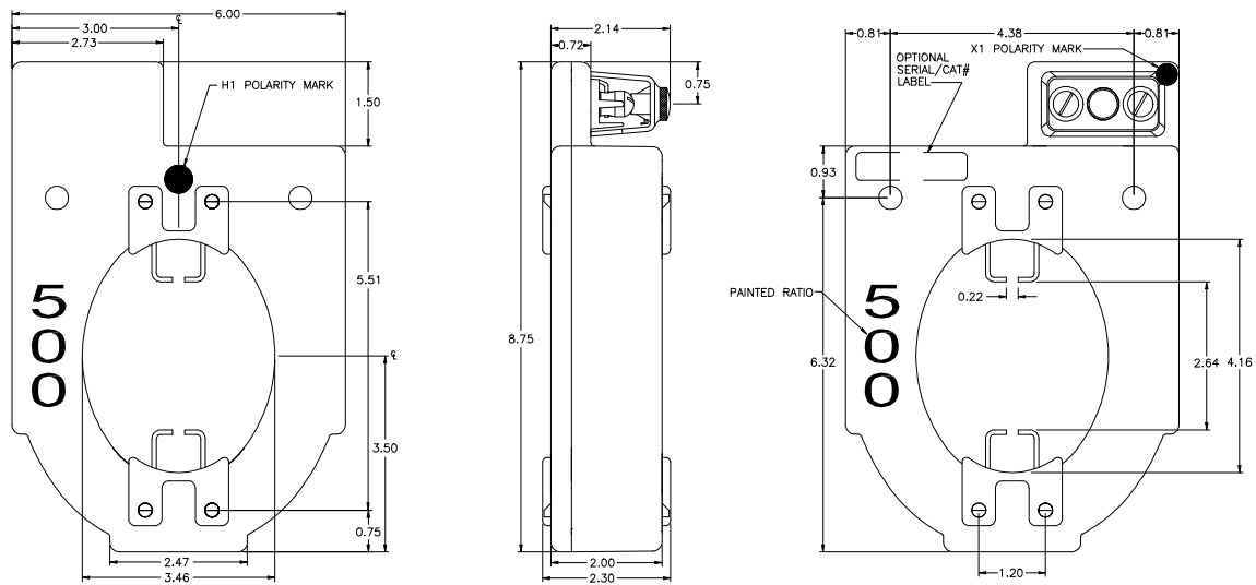
JAB-0W Dimensions
